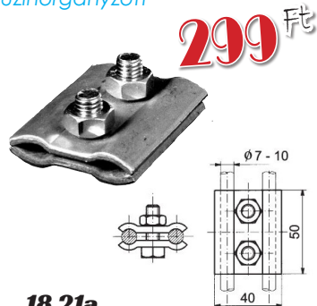
18 21a Fe / Zn tüzhorganyzott párhuzamos összekötő kapocs. Ø7-10, 50x40 mm
