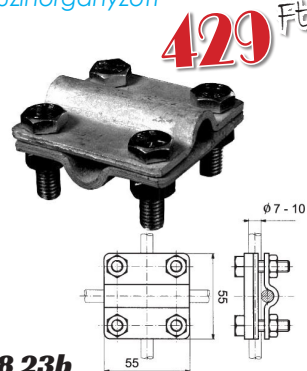
18 23b Fe / Zn tüzhorganyzott kereszt-kapocs. Ø7-10, 55x55 mm
