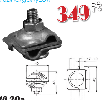
18 20a Fe / Zn tüzhorganyzott univerzális T alakú összekötő kapocs. Ø7-10, 45x45 mm
